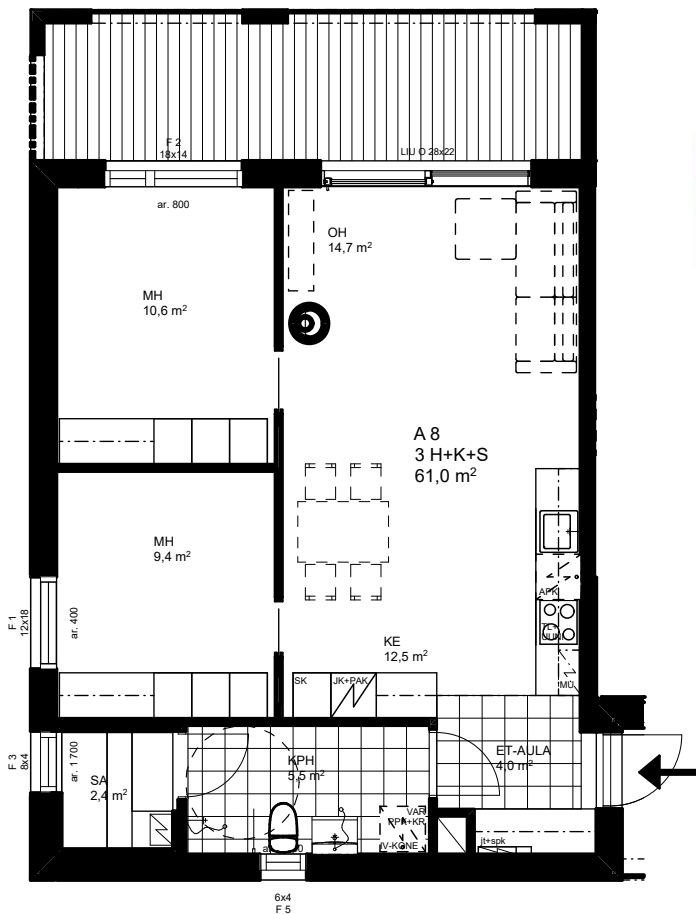
POHJAPIIRUSTUS 1:100
