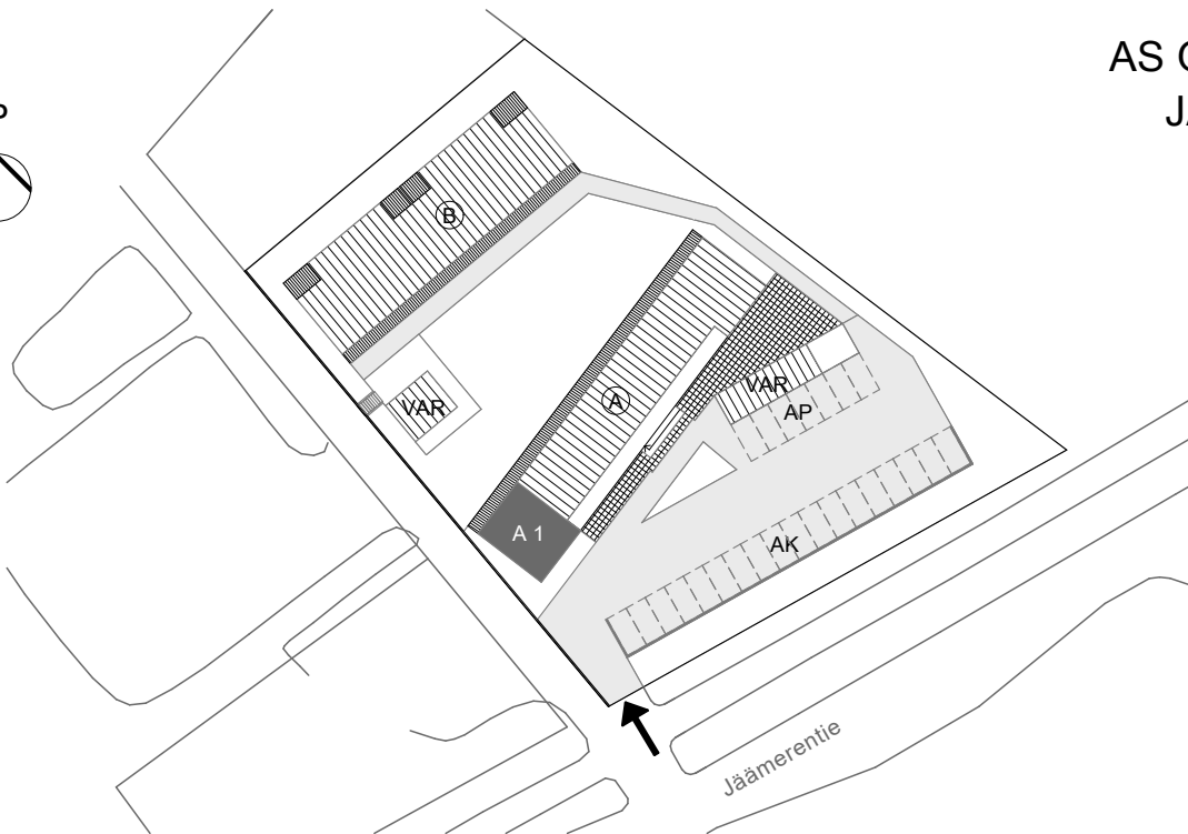
ASEMAPIIRUSTUS 1:1000
