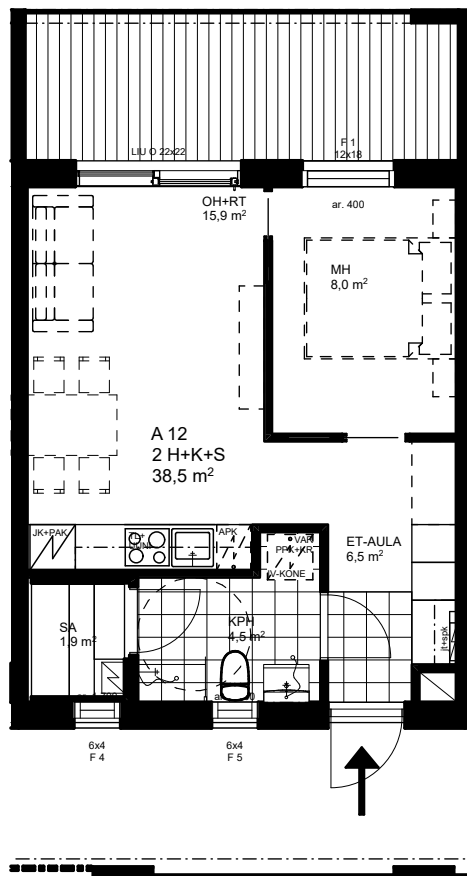
POHJAPIIRUSTUS 1:100
