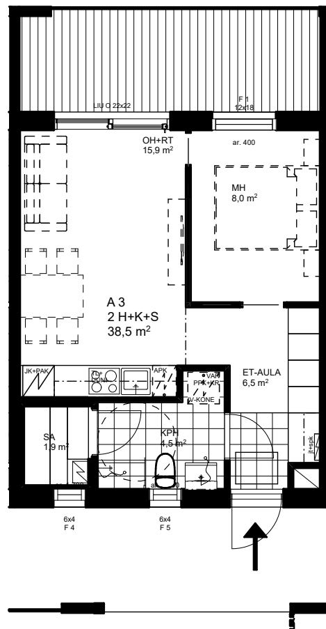
POHJAPIIRUSTUS 1:100
