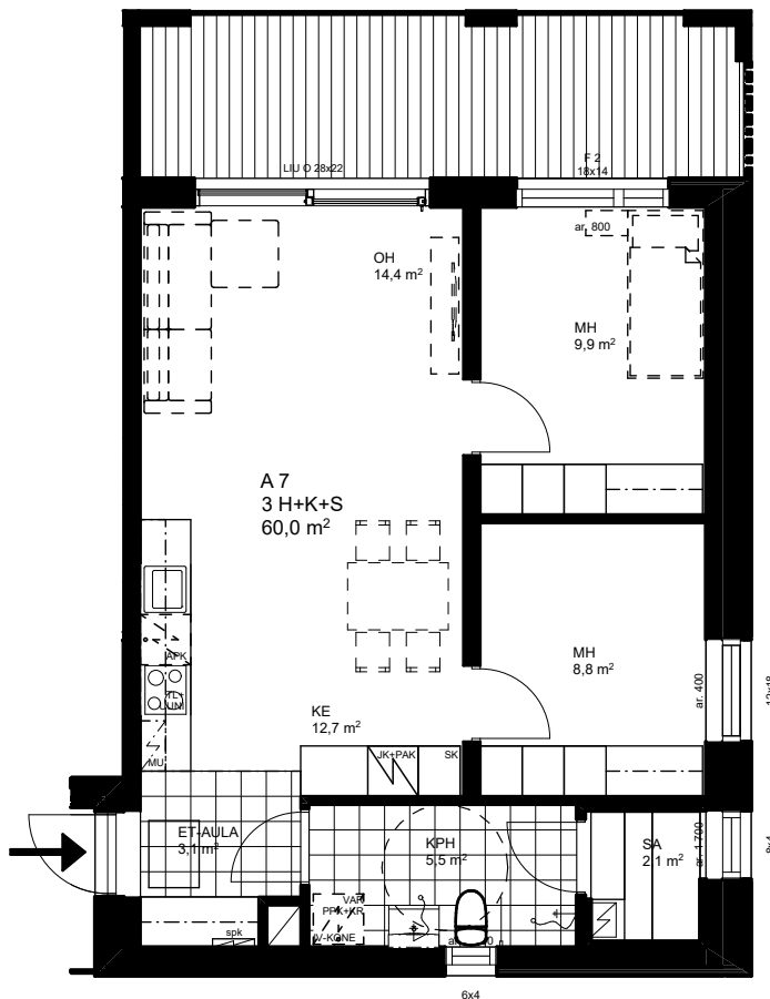
POHJAPIIRUSTUS 1:100
